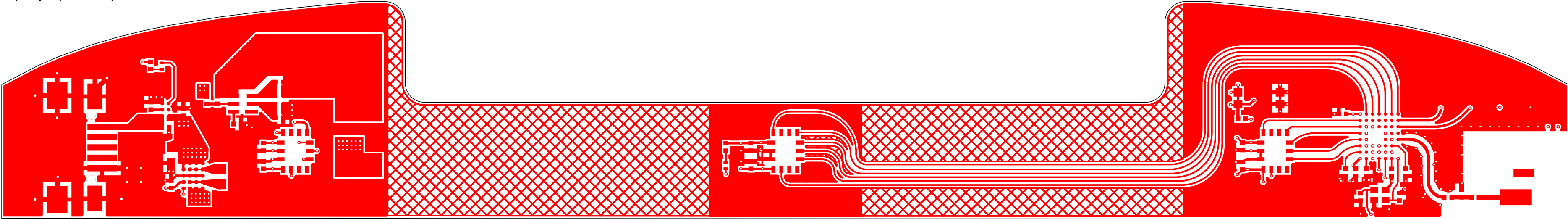
Top Layer (Scale 5:1)
