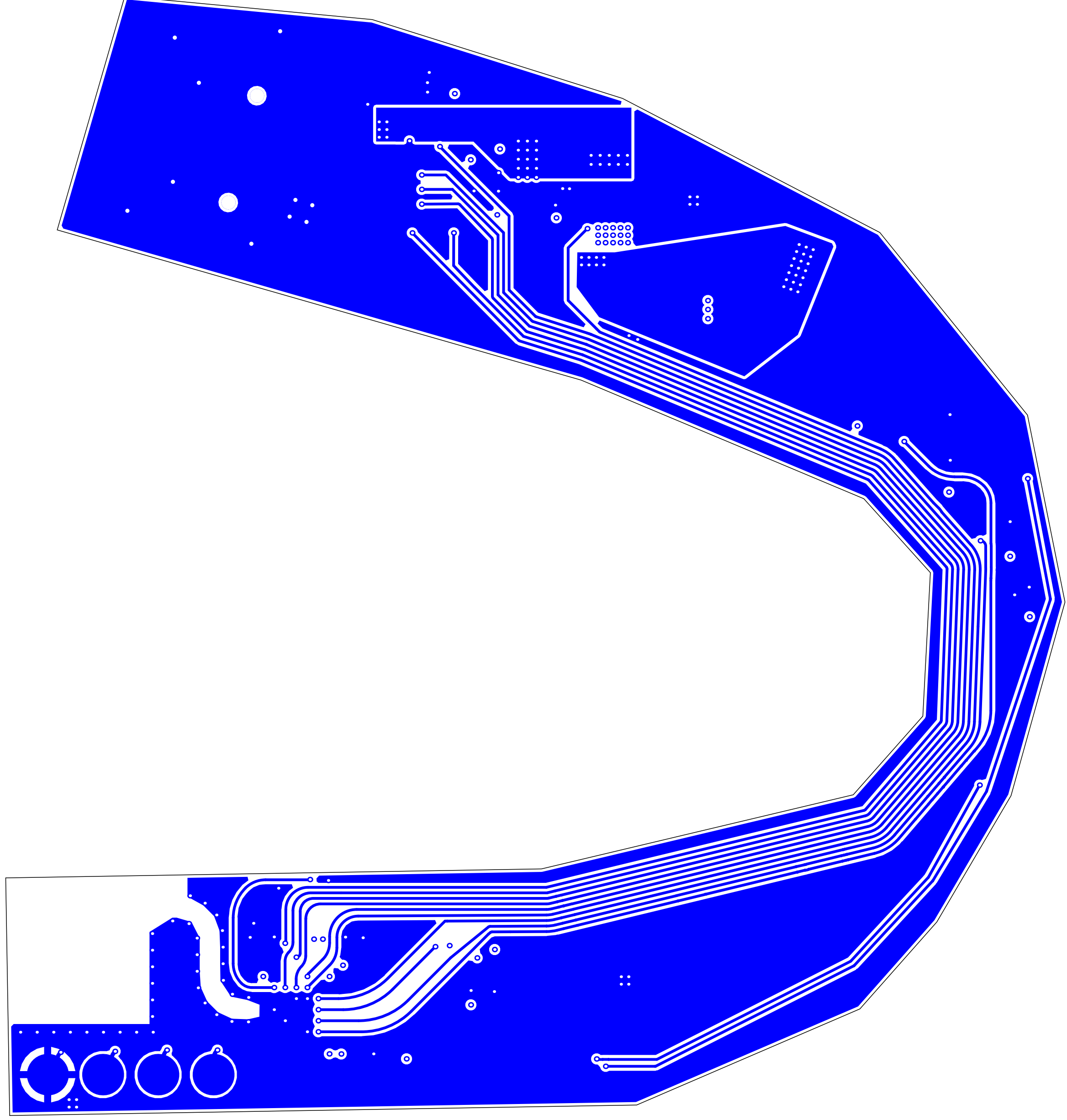
Bottom Layer (Scale 8:1)
