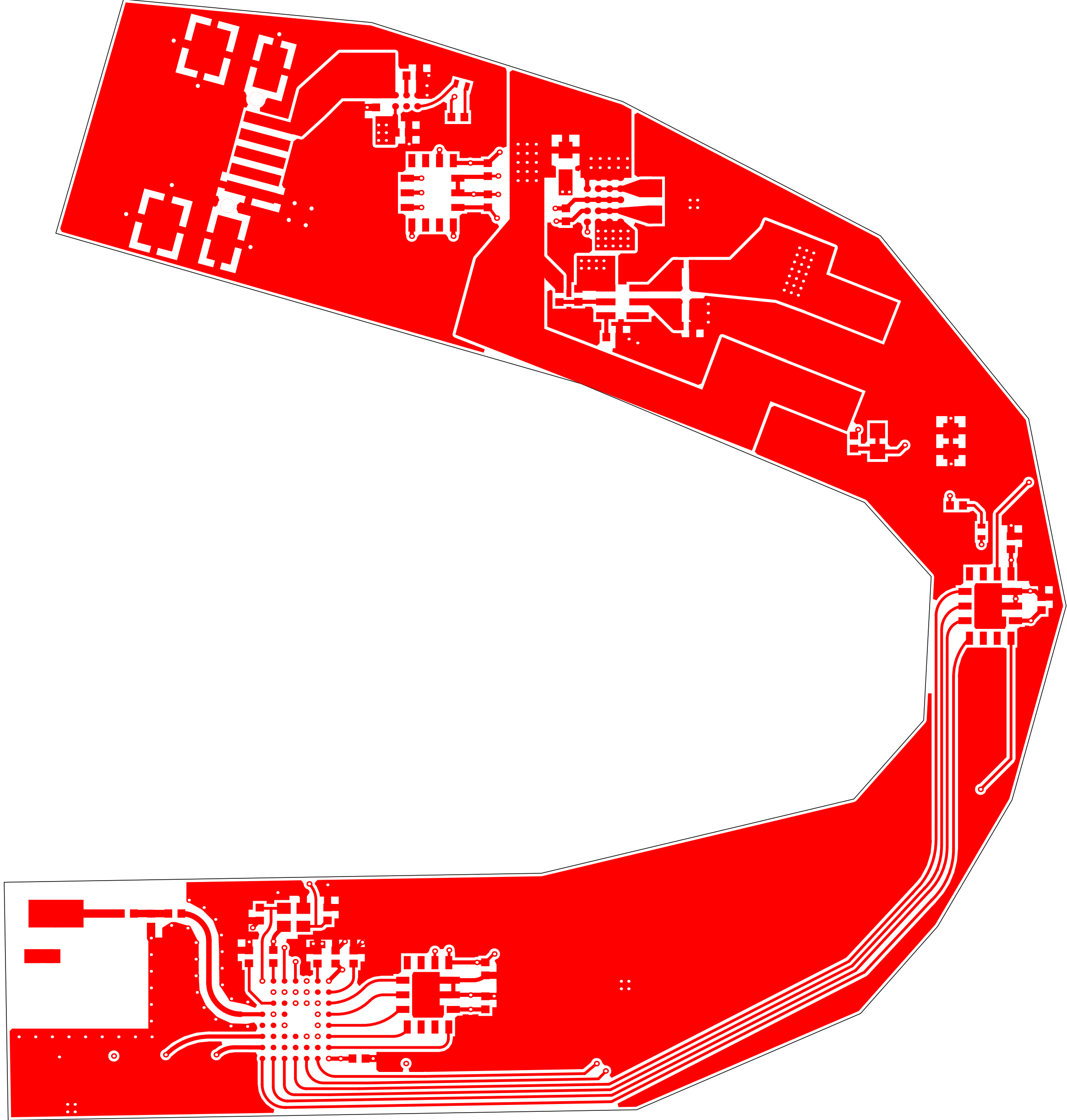
Top Layer (Scale 8:1)
