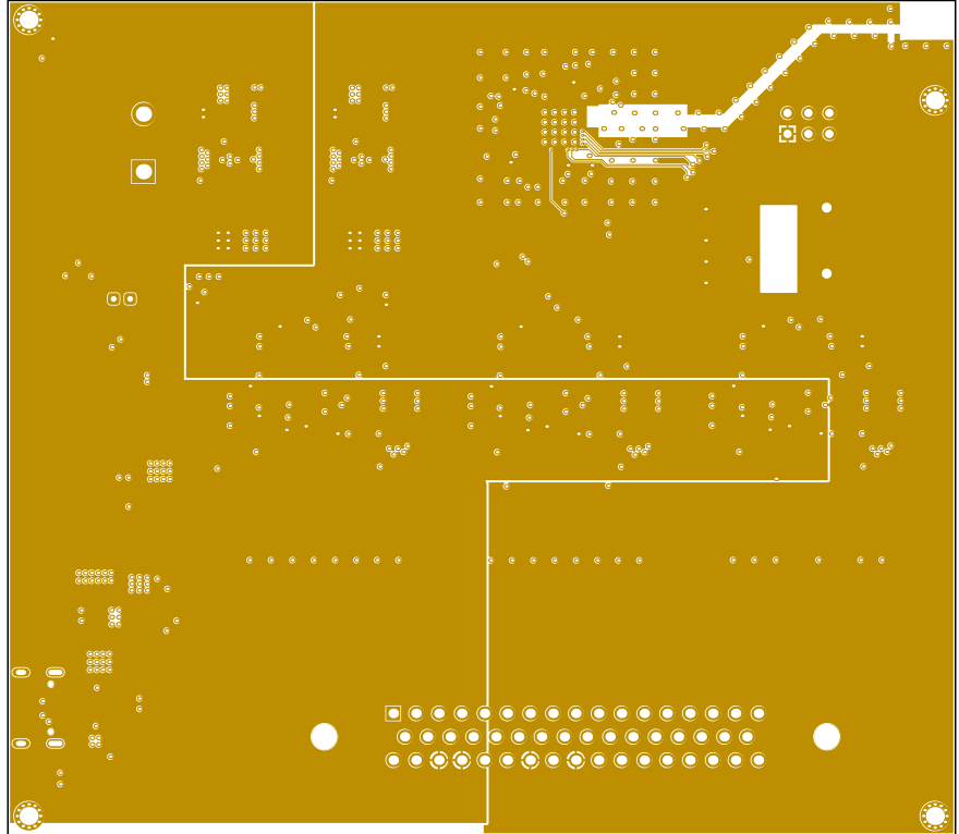
L2 - POWER (Scale 1:1)
