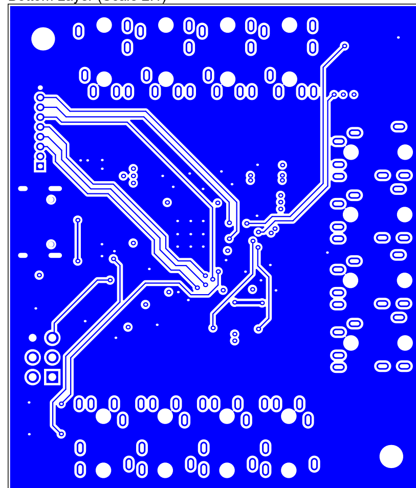
Bottom Layer (Scale 2:1)
