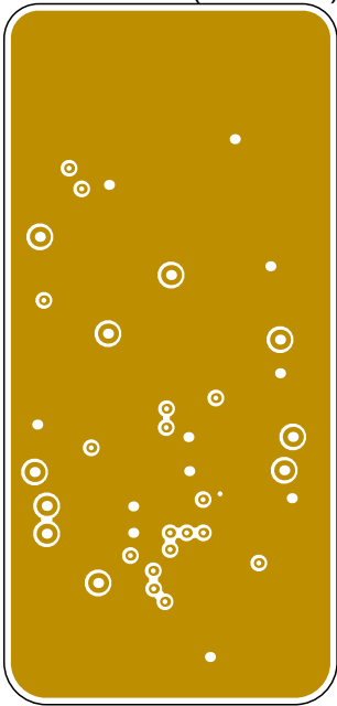
L2 - POWER (Scale 4:1)
